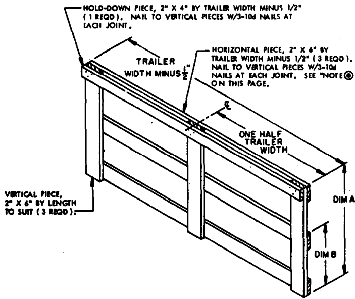
REAR OF LOAD GATE (D)
